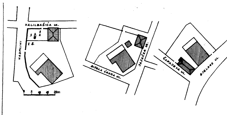
Sl. 25. Situacije nekih mekteba u Sarajevu
