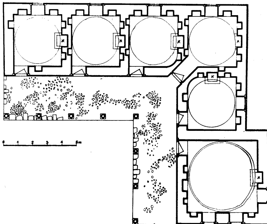
Sl. 58. Medresa Šišman Ibrahim paše u Počitelju, tlocrt
