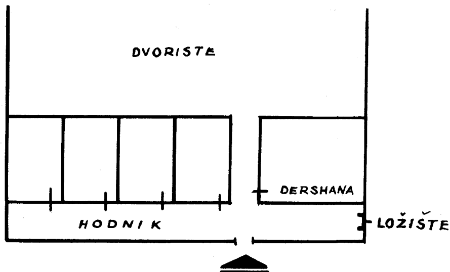
Sl. 91. Medresa uz Jeni džamiju u Preševu, skica tlocrta
