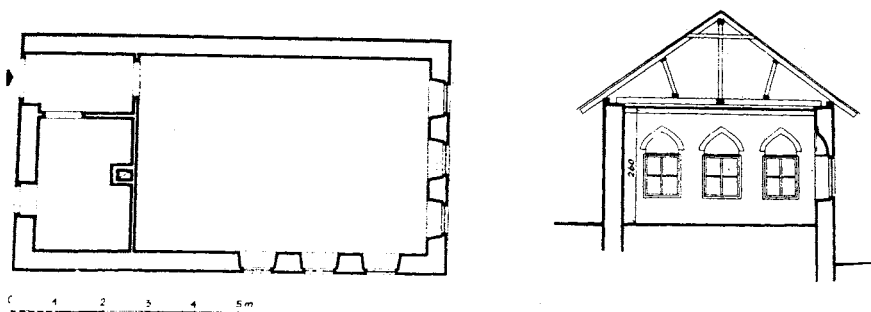
Sl. 35. Mekteb uz džamiju Nebrdilo Hadži Alije u Sarajevu, tlocrt i presjek
