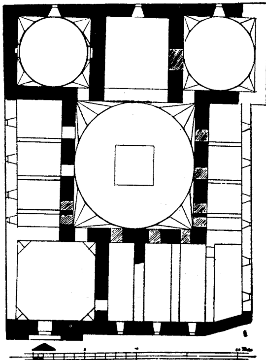
Sl. 3. Karataj medresa u Konji, tlocrt
