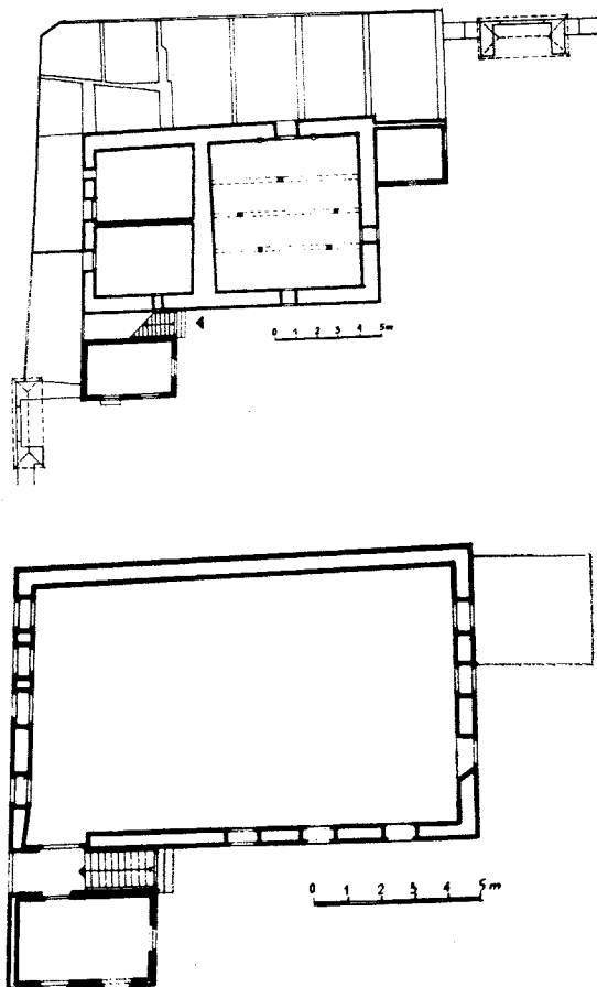
Sl. 32. Gazi Husrevbegov mekteb u Sarajevu, tlocrt prizemlja i kata
