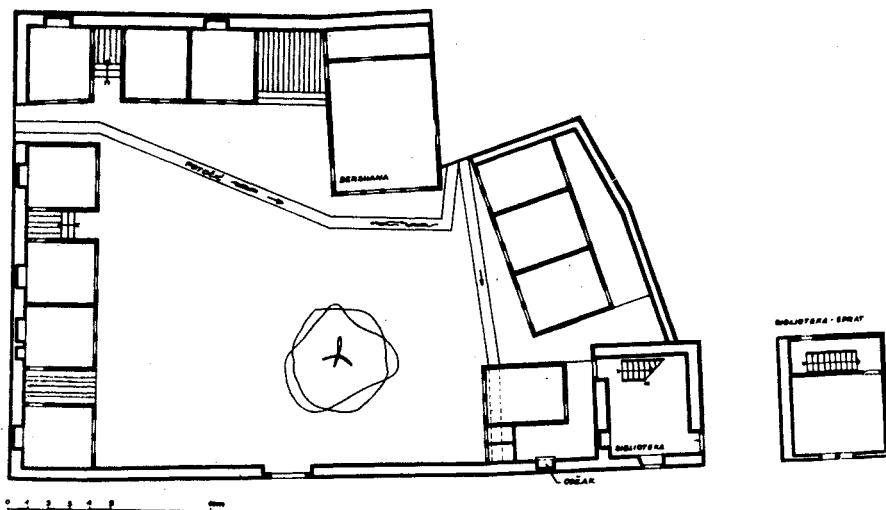
Sl. 92. Atik medresa u Peći, tlocrt
