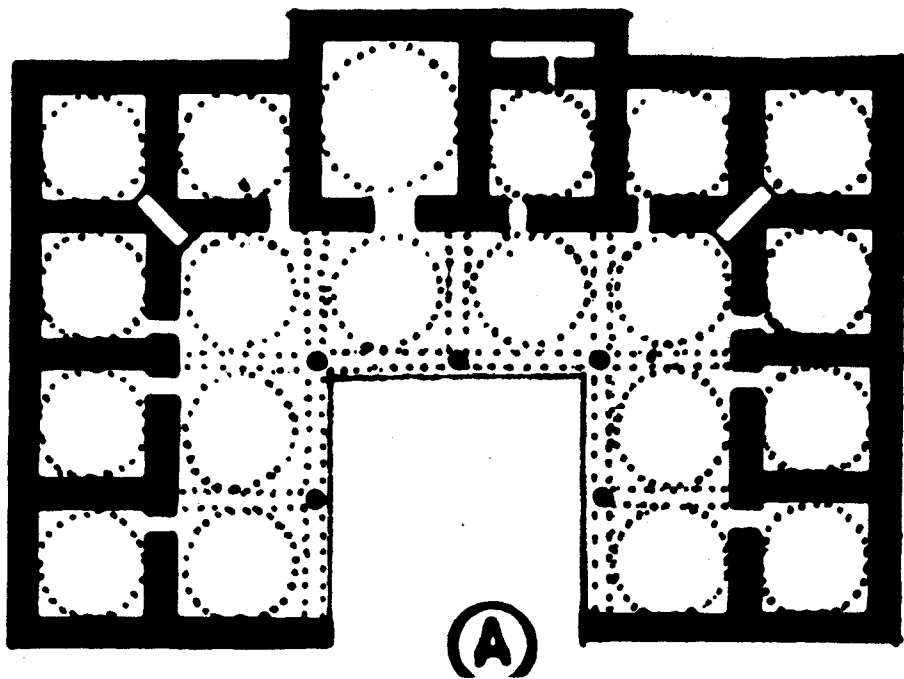
Sl. 13. Medresa Sulejman-paše u Izniku, tlocrt
