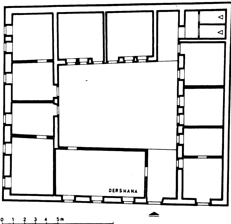
Sl. 52. Medresa u Konjicu u blizini Junuz Čauš džamije, tlocrt
