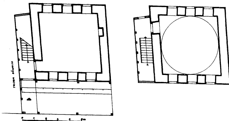
Sl. 99. Biblioteka uz Hadim džamiju u Đakovici, tlocrt prizemlja i kata
