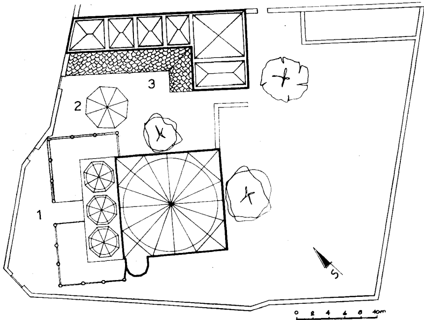
Sl. 63. Karadžobegova medresa u Mostaru, situacija
