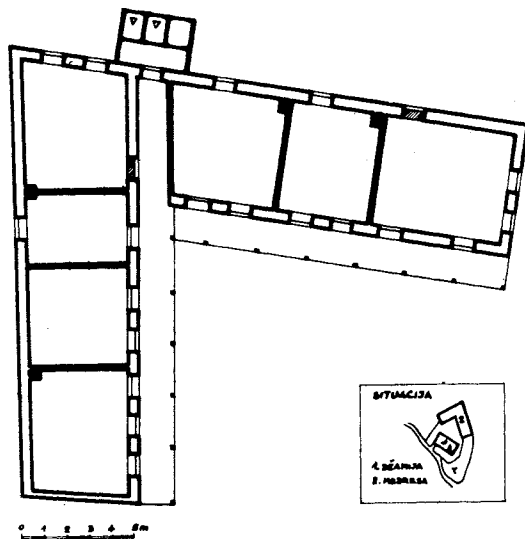
Sl. 73. Medresa Mehmed paše Muhsinovića u Travniku (Lončarica), tlocrt
