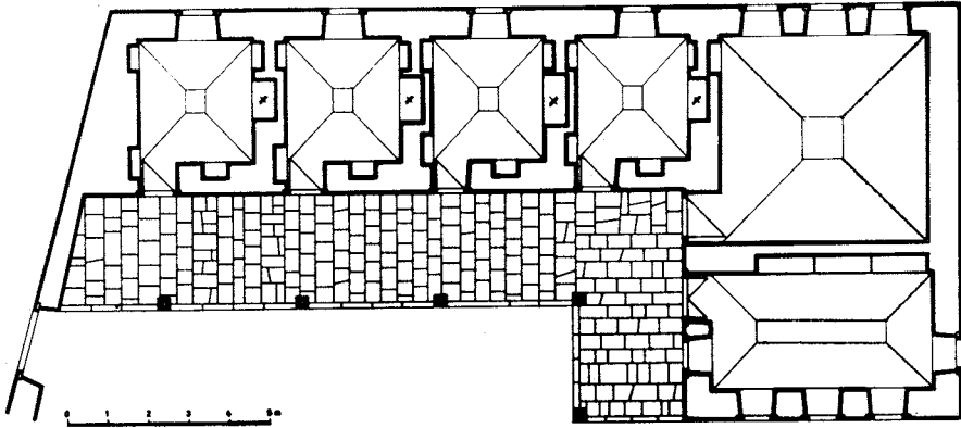
Sl. 64. Karadžbegova medresa u Mostaru, tlocrt
