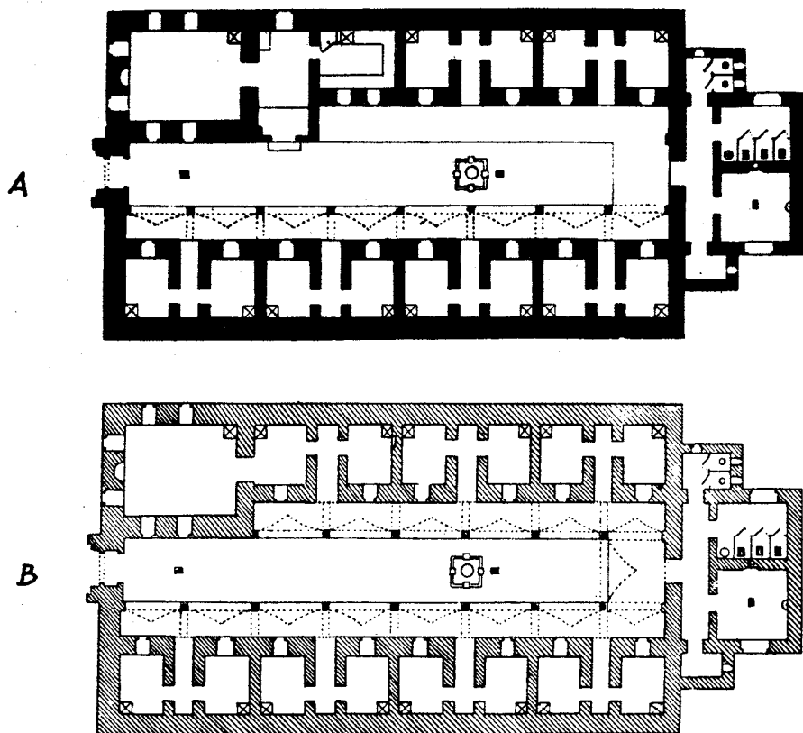
Sl. 50. Gazi Husrevbegov hanikah u Sarajevu, tlocrt A. stanje iz 1912. godine, B. rekonstrukcija
