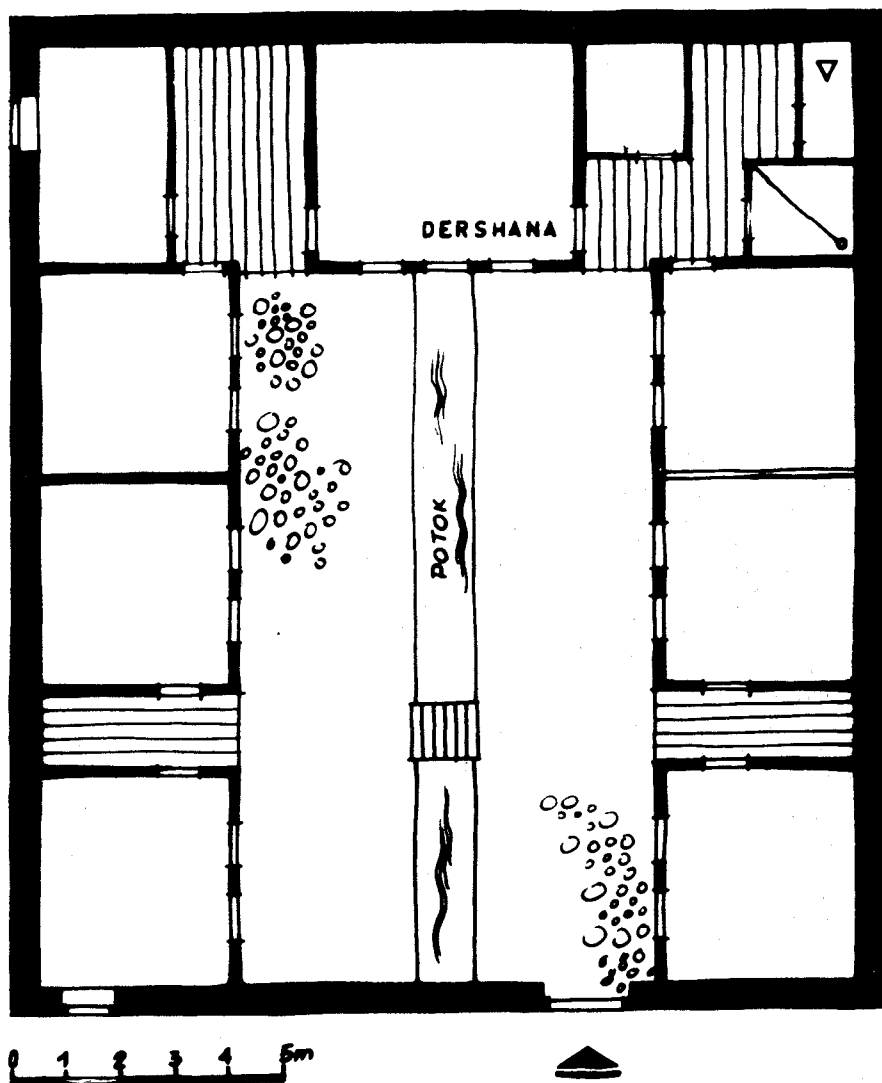
Sl. 53. Medresa u Žepču, rekonstrukcija tlocrta
