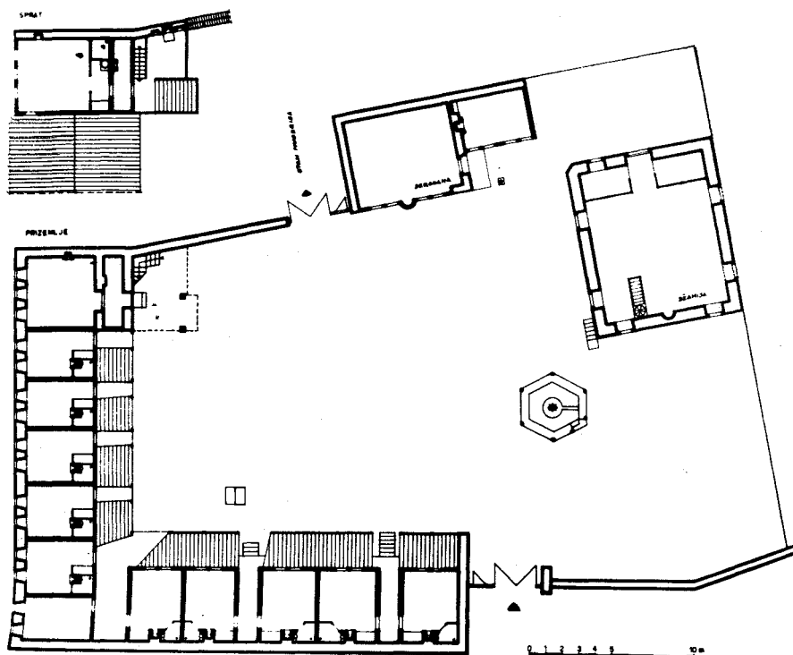
Sl. 94. Velika medresa u Đakovici, tlocrt
