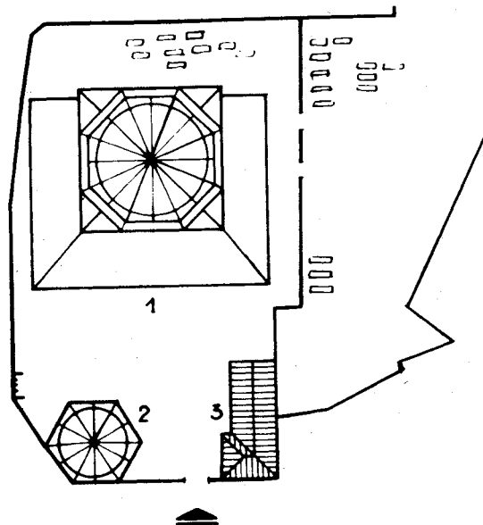
Sl. 82. Biblioteka Osman Šuhdije u Sarajevu, situacija 1. Careva džamija 2. biblioteka 3. muvekithana
