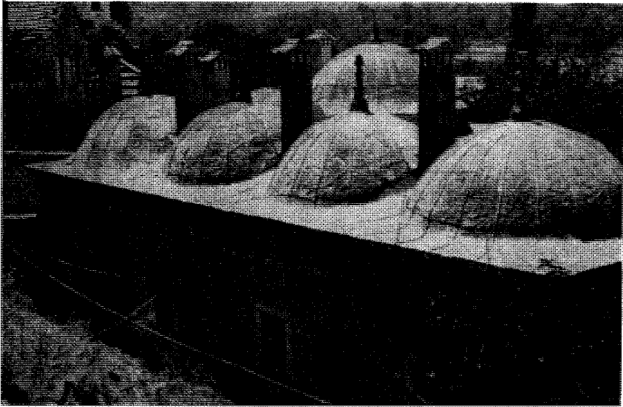
Sl. 62. Medresa Šišman Ibrahim paše u Počitelju, izgled
