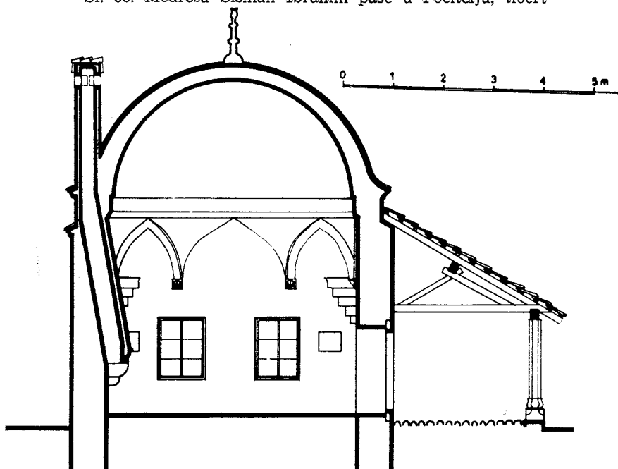
Sl. 59. Medresa Šišman Ibrahim paše u Počitelju, presjek
