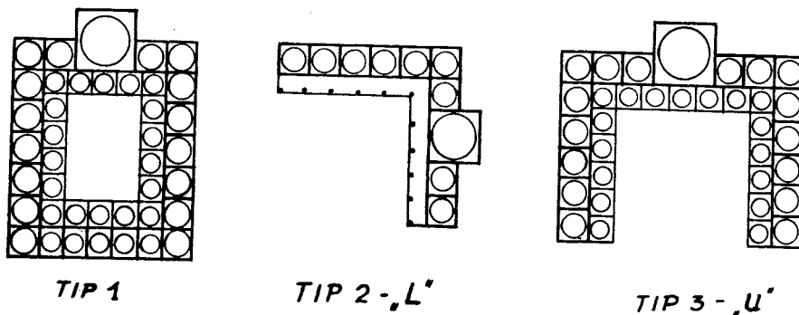
Sl. 16. Šeme osnovnih tipova osmanskih medresa
