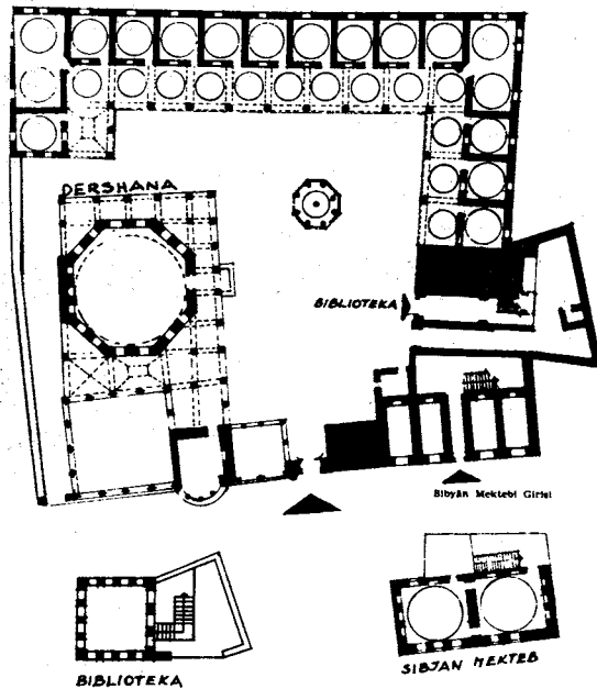
Sl. 21. Medresa Amdža zade Husein-paše u Carigradu, tlocrt
