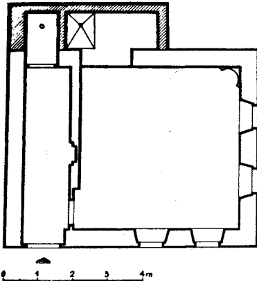
Sl. 28. Mekteb uz džamiju Kučuk katib Muhjudina u Sarajevu, tlocrt i presjek
