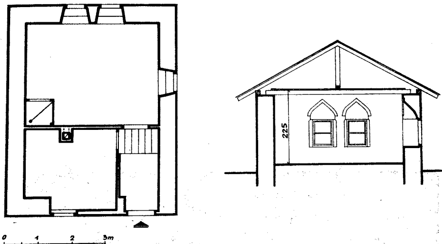
Sl. 33. Mekteb Divan katib Hajdar efendije u Sarajevu, tlocrt i presjek
