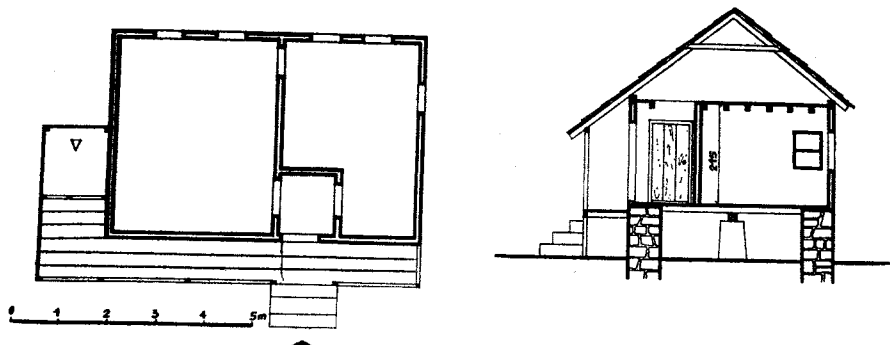
Sl. 39. Dvojni mekteb kod Konatur džamije u Travniku, tlocrt i presjek
