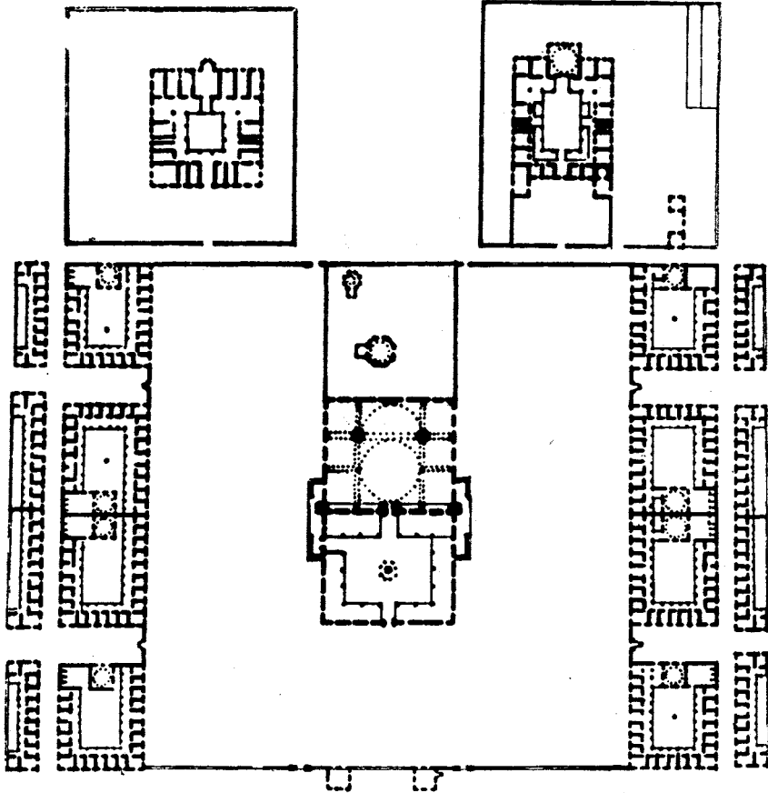
Sl. 19. Kompleks Fatihove džamije u Carigradu, tlocrt
