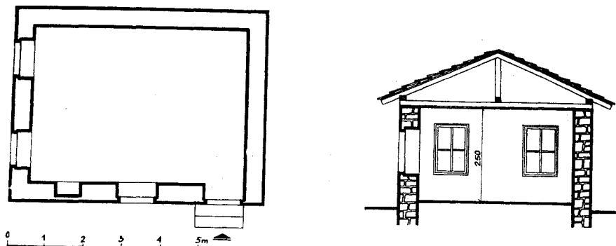
Sl. 26. Mekteb uz Cerničku džamiju u Mostaru, tlocrt i presjek
