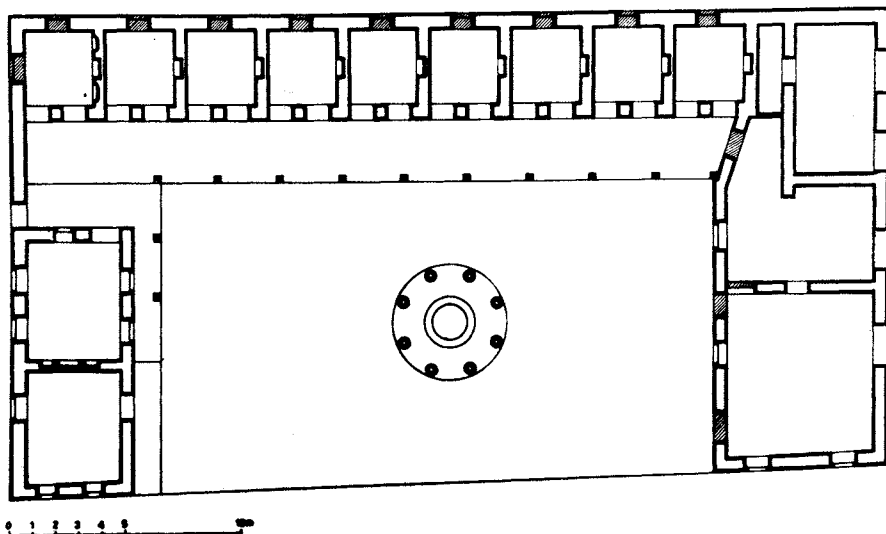
Sl. 70. Medresa Roznamedži Ibrahim-efendije u Mostaru, tlocrt
