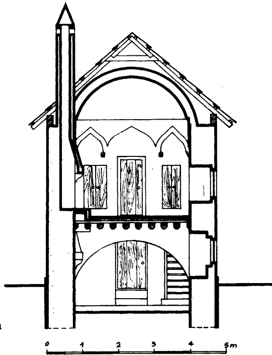
Sl. 79. Medresa i tekija Hasan Kafi ef. u Pruscu, presjek
