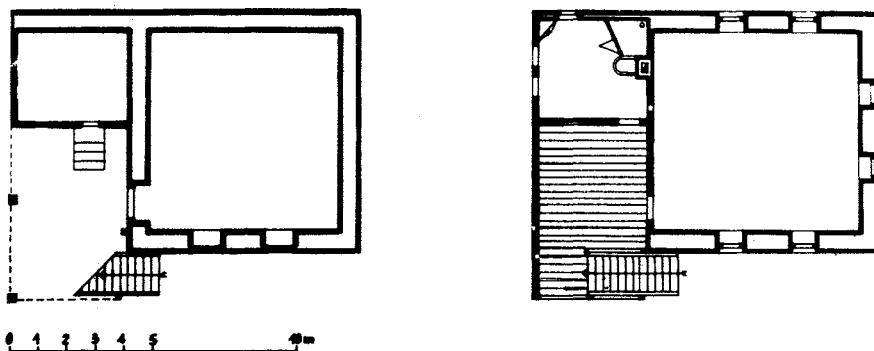
Sl. 37. Mekteb uz Altun alem džamiju u Novom Pazaru, tlocrt prizemlja i kata
