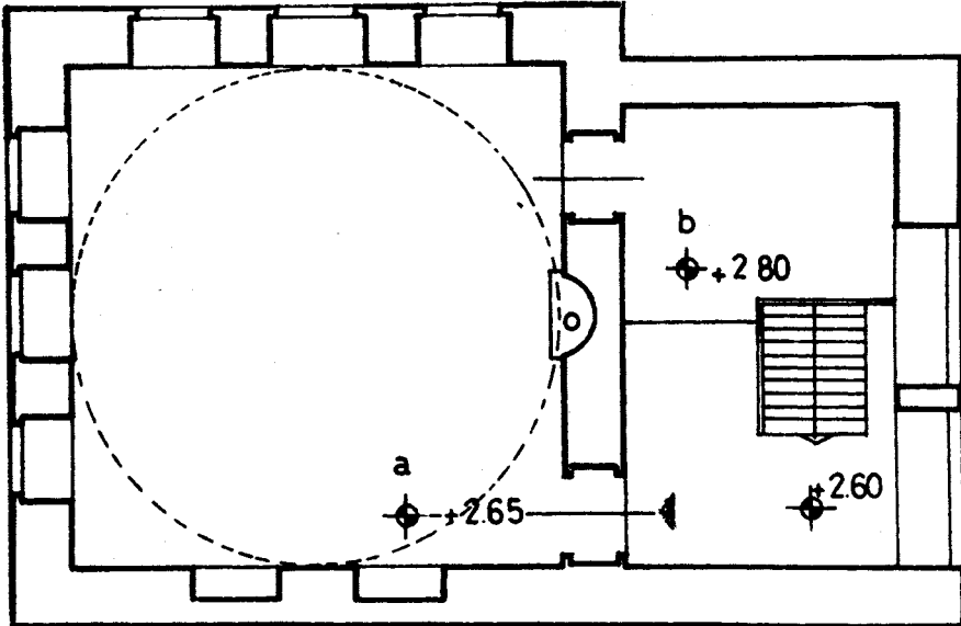
Sl. 8. Tavšant mekteb u Carigradu, tlocrt
