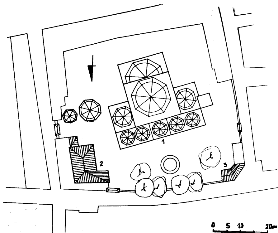
Sl. 31. Mekteb Gazi Husrevbega u Sarajevu, situacija: 1. džamija, 2. mekteb, 3. muvekitihana
